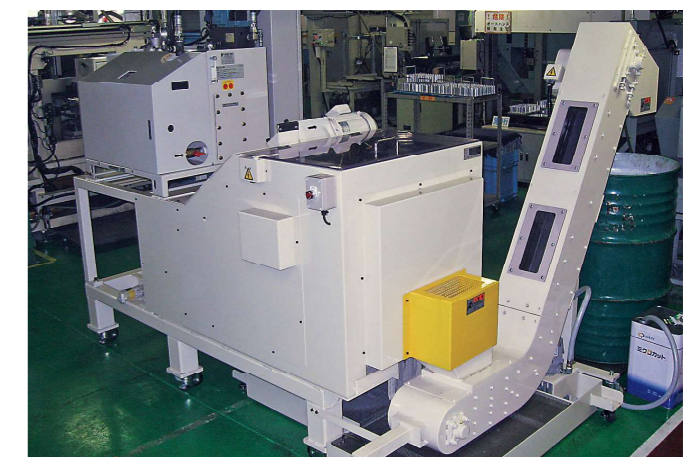
■設置例 切粉圧縮機 SPS-40SYR
