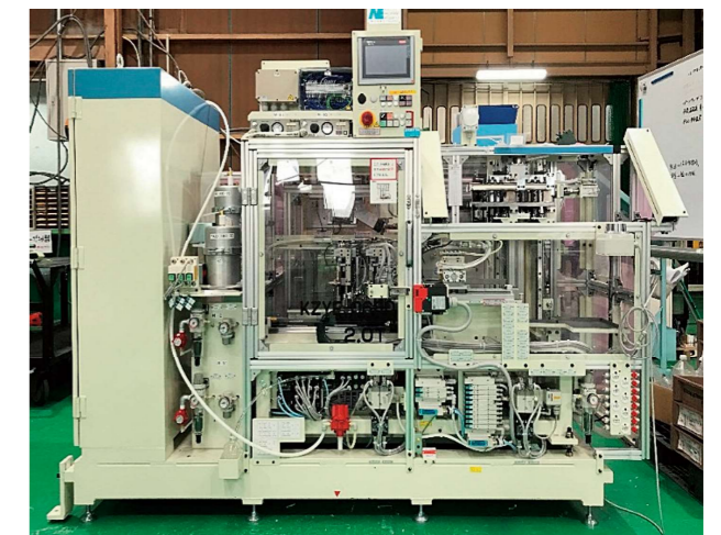
複合組付グリス塗布機
