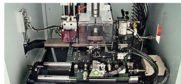
タップ加工 (専用機)
